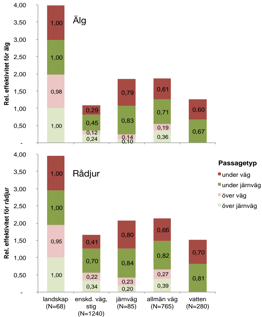
Figur 42. Passagerans relativa effektivitet för älg uppdelat på över- och undergångar vid väg- och järnvägsbarriärer. N = 2438.
